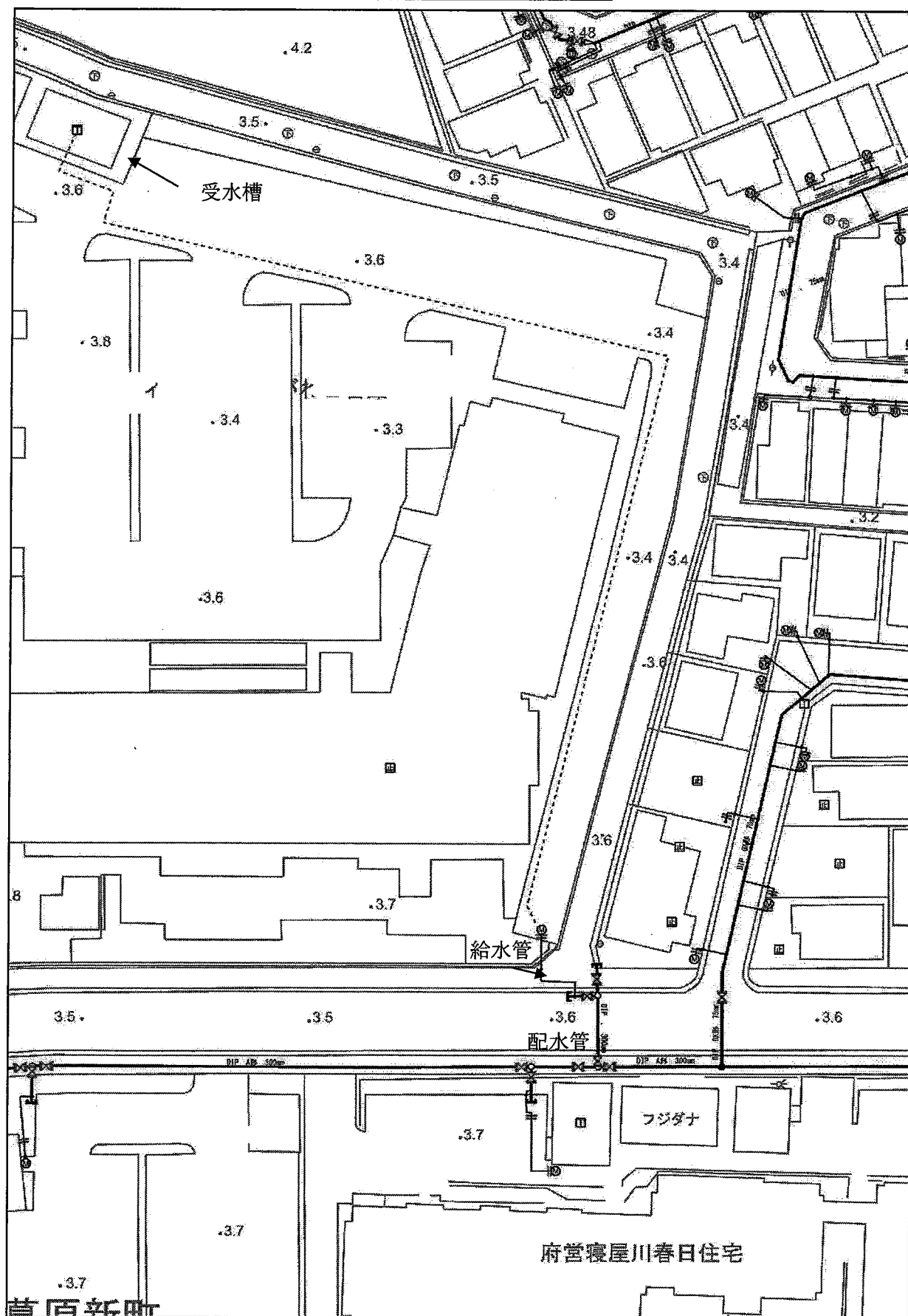
水道施設台帳図
