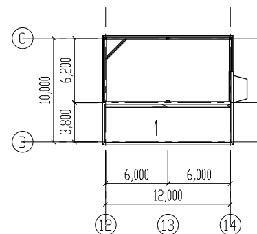
PHR階平面図
