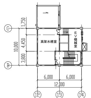
PH 1階平面図
