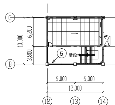
PH 2階平面図
