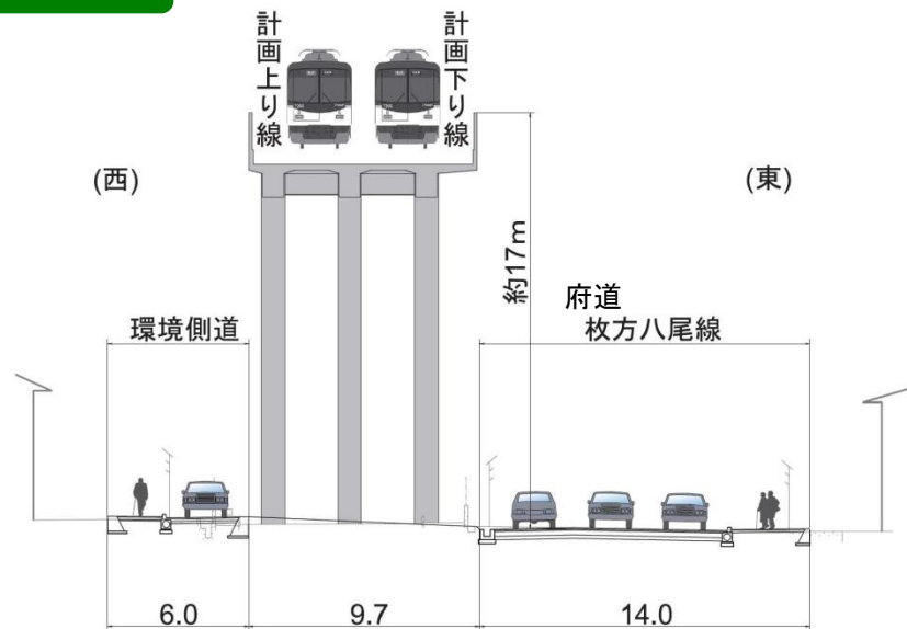
B-B'断面図
