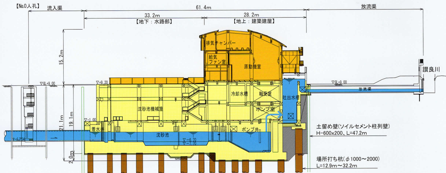
縦断面図 ①-①
