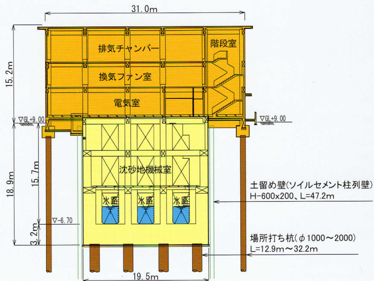
横断面図 ②-②
