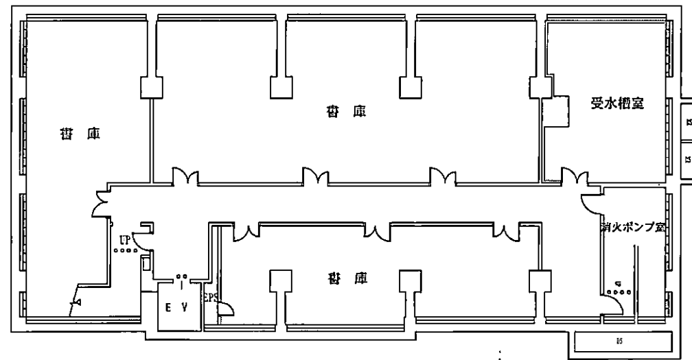
議会棟地下一階平面図
