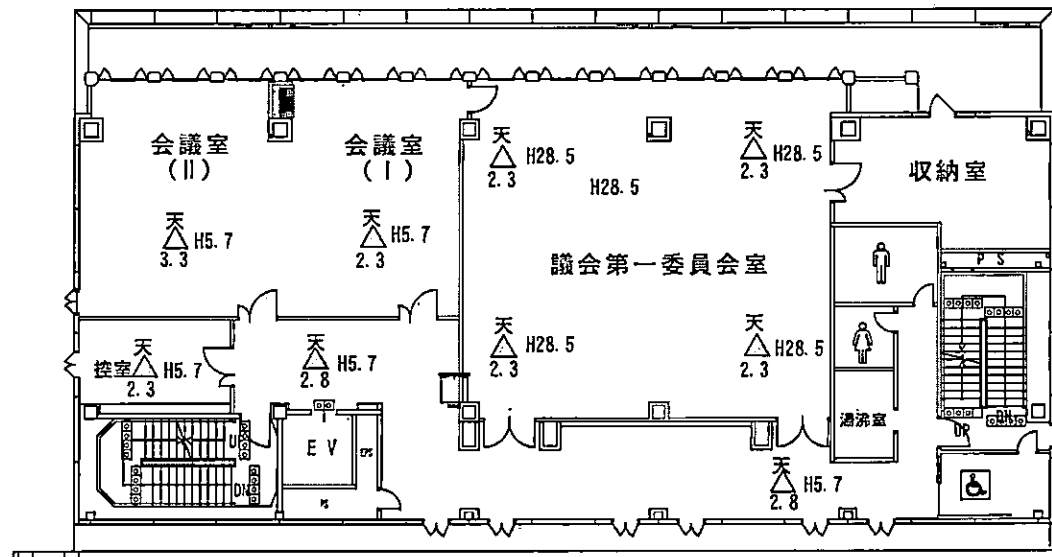
議会棟四階平面図
