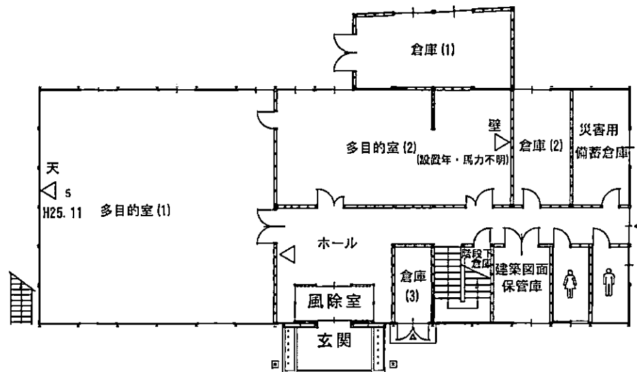
別館一階平面図
