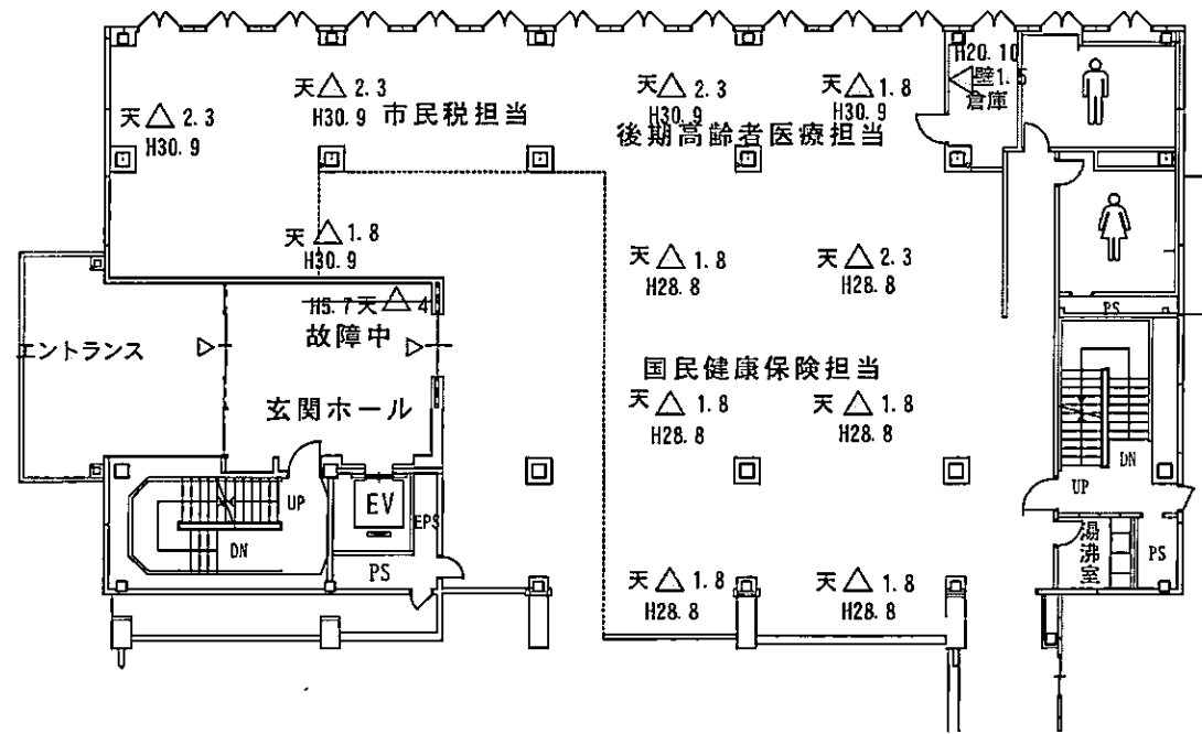
議会棟一階平面図
