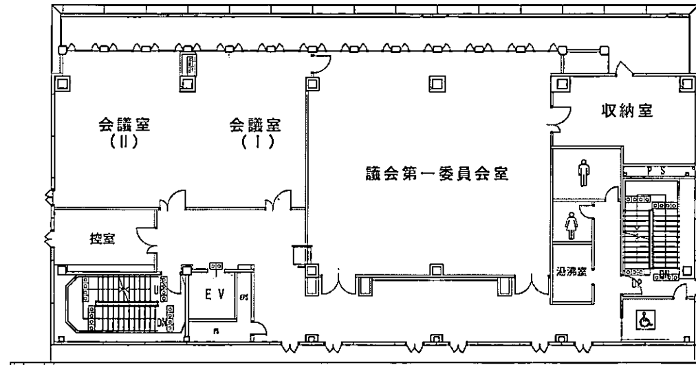
議会棟四階平面図
