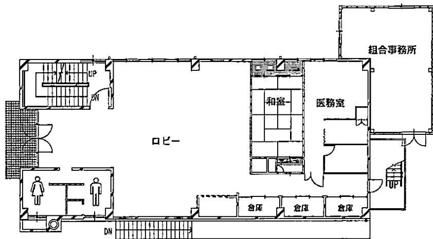
一階平面図
