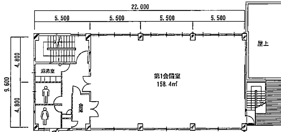
三階平面図
