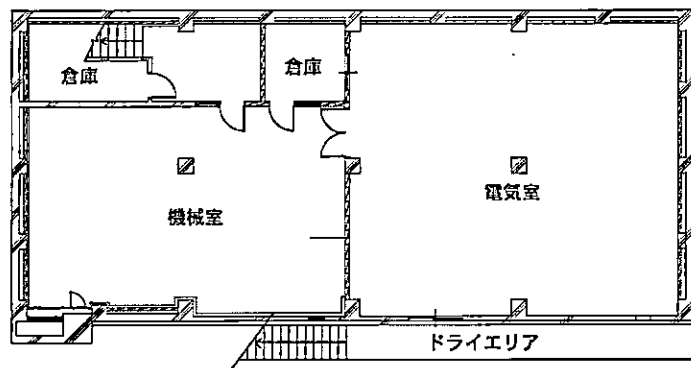
地下一階平面図
