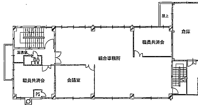
二階平面図
