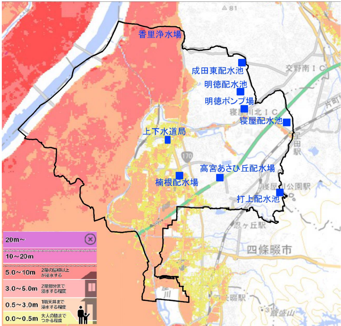
图 2-19 洪水氾滥浸水位
