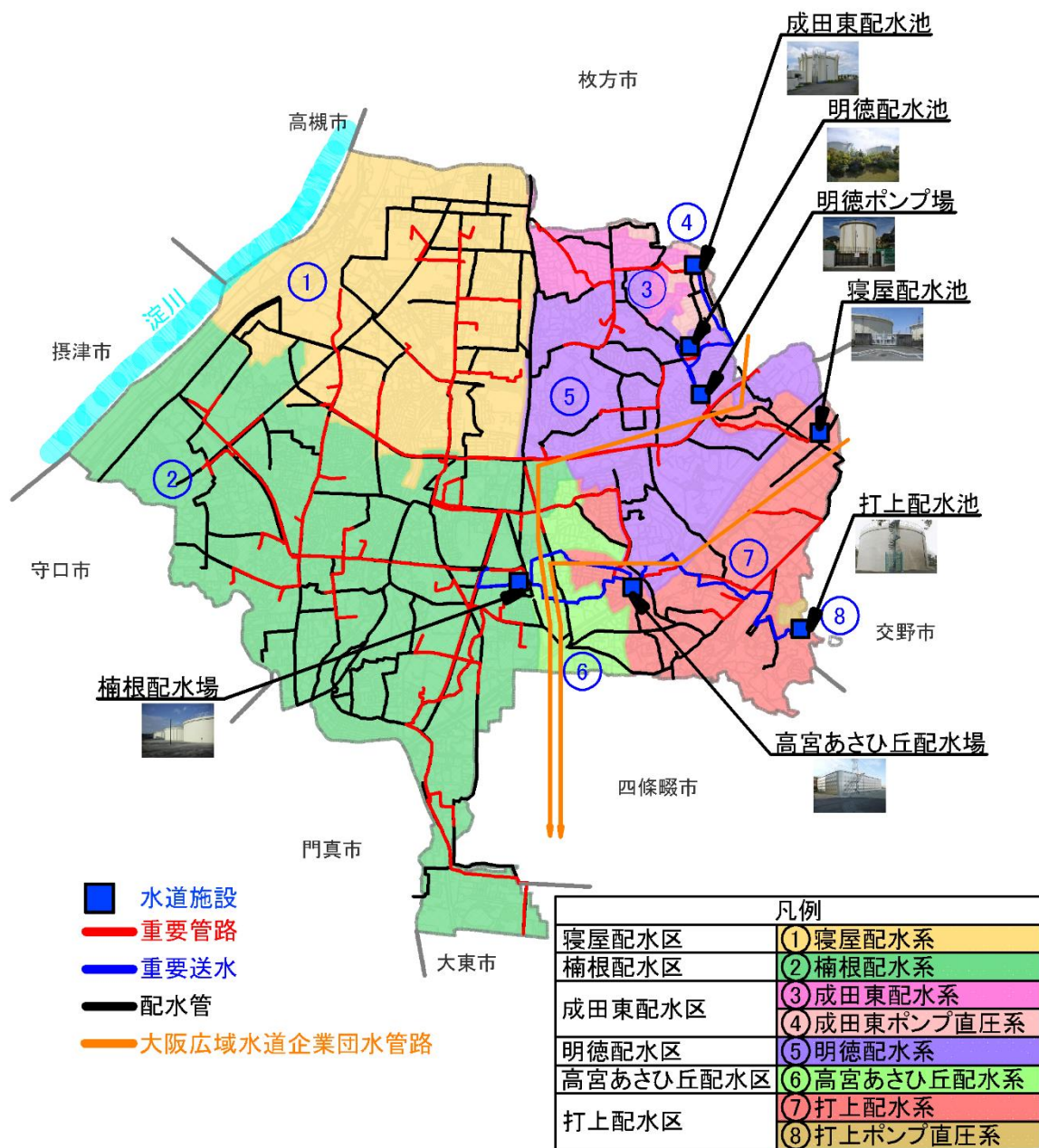
図 2-24 配水区域と水道施設及び管路等の平面図
