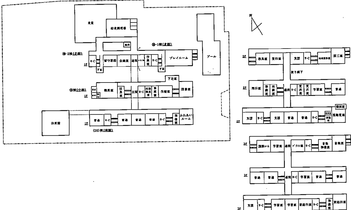
明和小学校 配便・平面図
