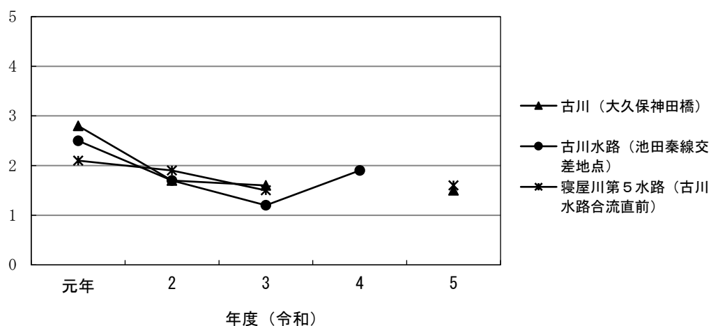
図 2.2.3 古川水系における生物化学的酸素要求量（平均値）の推移
