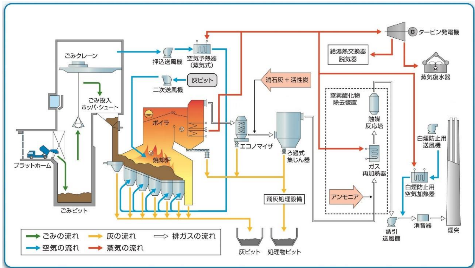
図 3.3.1 可燃ごみの処理
