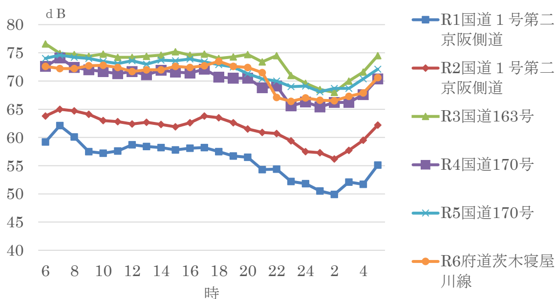
図 2-3. 2. 1 道路騒音経時変化 (L Aeq )
