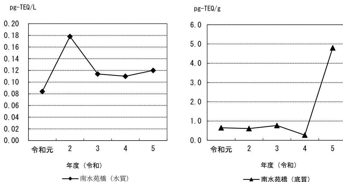
図 2-5. 2. 2 ダイオキシン類濃度測定結果（河川）の推移
