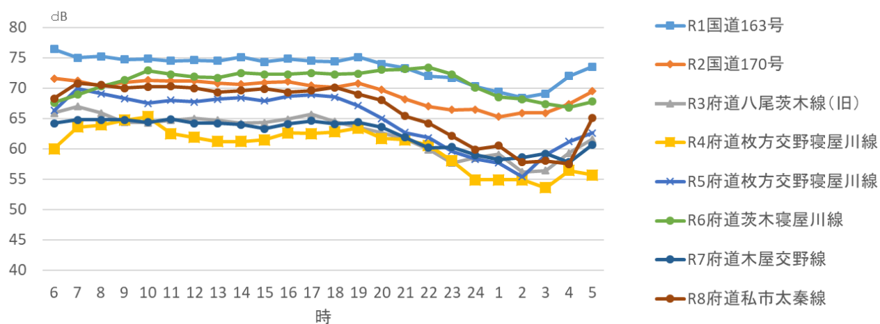
図 2-3.2.1 道路騒音経時変化 (L Aeq )
