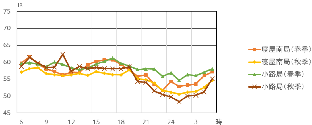
図 2-3. 2. 5 道路騒音経時変化 (L Aeq )
