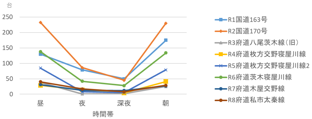
図 2-3. 2. 3 10 分間交通量の変化
