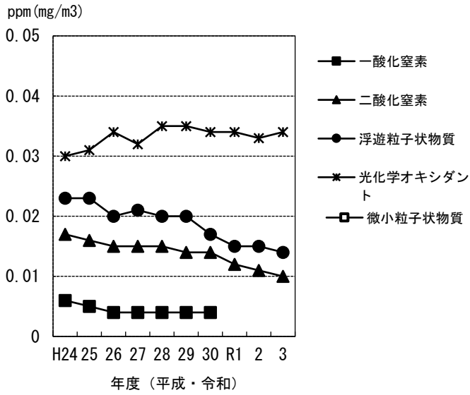
図 2-1.2.1 大気汚染測定結果の推移（寝屋川市役所局）
