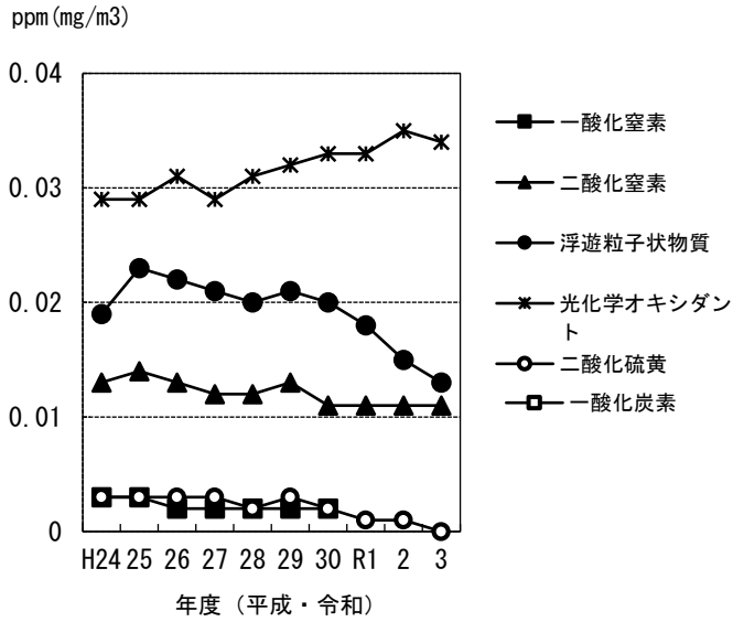
図 2-1.2.2 大気汚染測定結果の推移（成田局）
