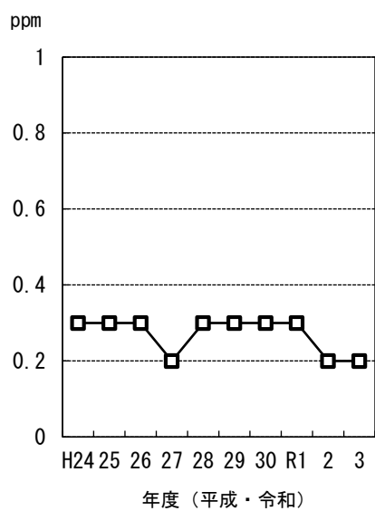
図 2-1.2.2 大気汚染測定結果の推移（成田局）
