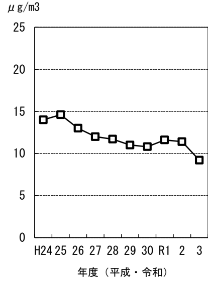
図 2-1.2.1 大気汚染測定結果の推移（寝屋川市役所局）
