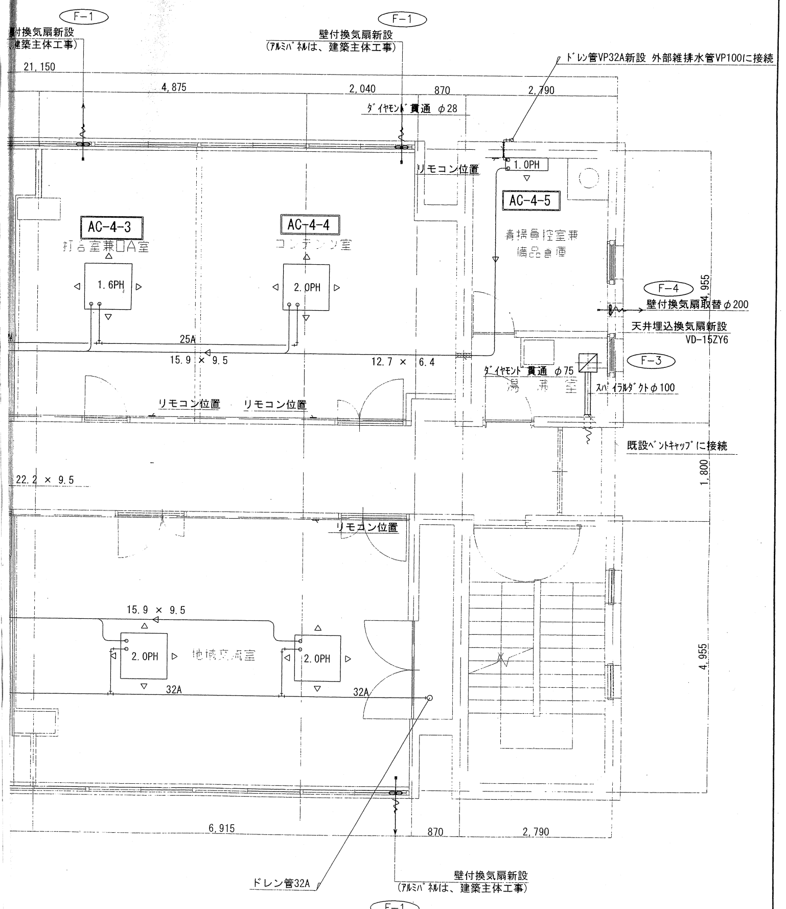
4 階 平 面 図
