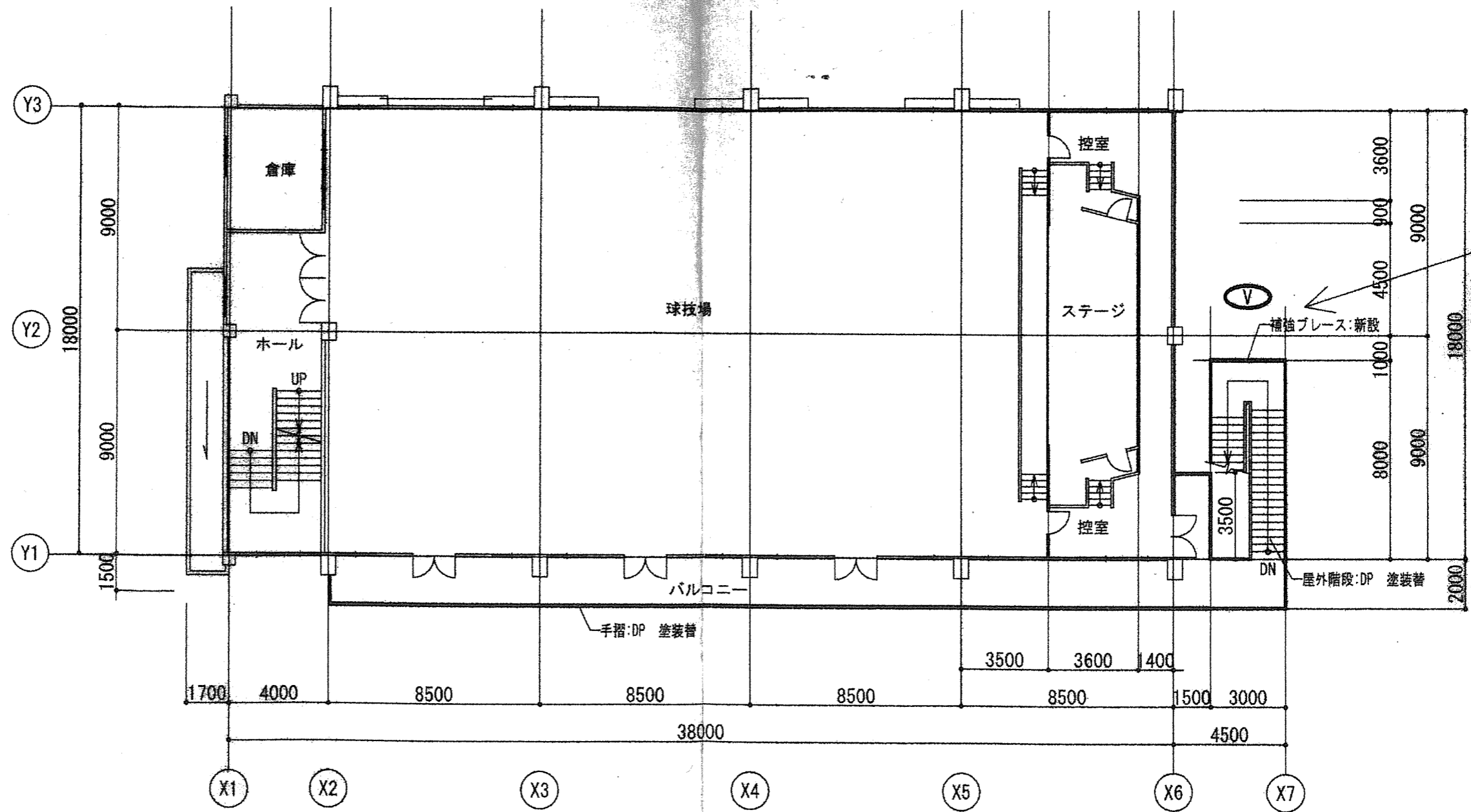
2 階 平面図
